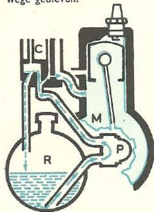
P brandstofpompje R brandstoftank C carburateur M motor
