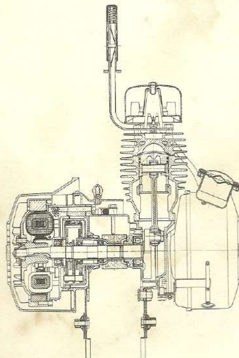
Doorsnede van de Solexmotor
